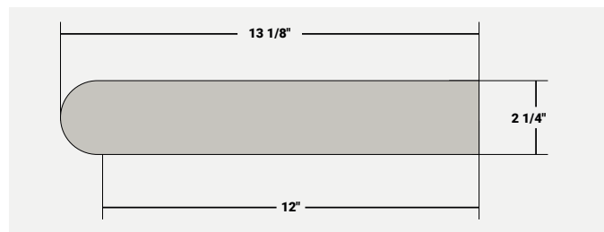
REBORD ARRONDI
