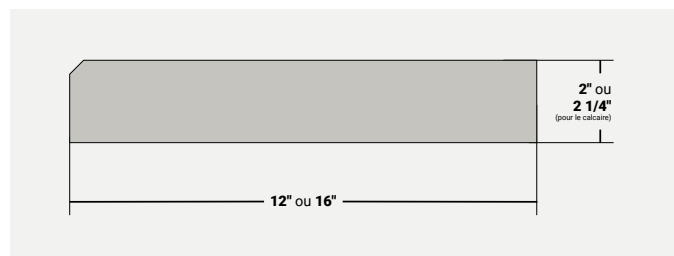
REBORD CHANFREINÉ
